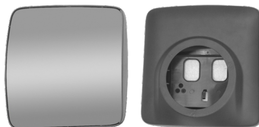
RETROVISOR AUXILIAR VOLVO FH 2015 C/ DESEMBAÇADOR ELETRICO LE/LD APLICAÇÃO: VOLVO FH 2015 EM DIANTE CÓDIGO PRODUTO: 0060054 CODIGO FÁBRICA: ER1258
